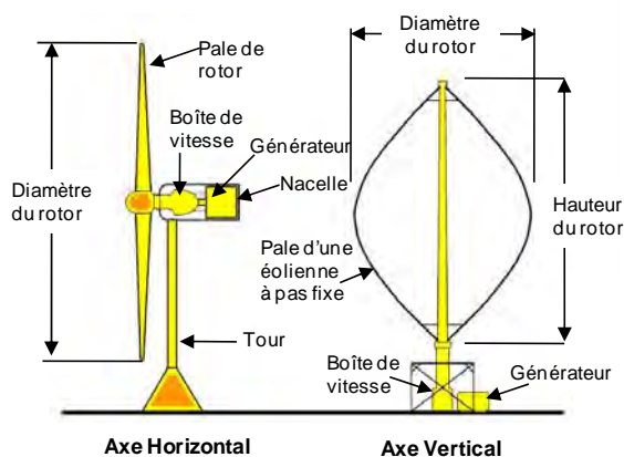
Figure 1. Configuration typique d'une éolienne 1
