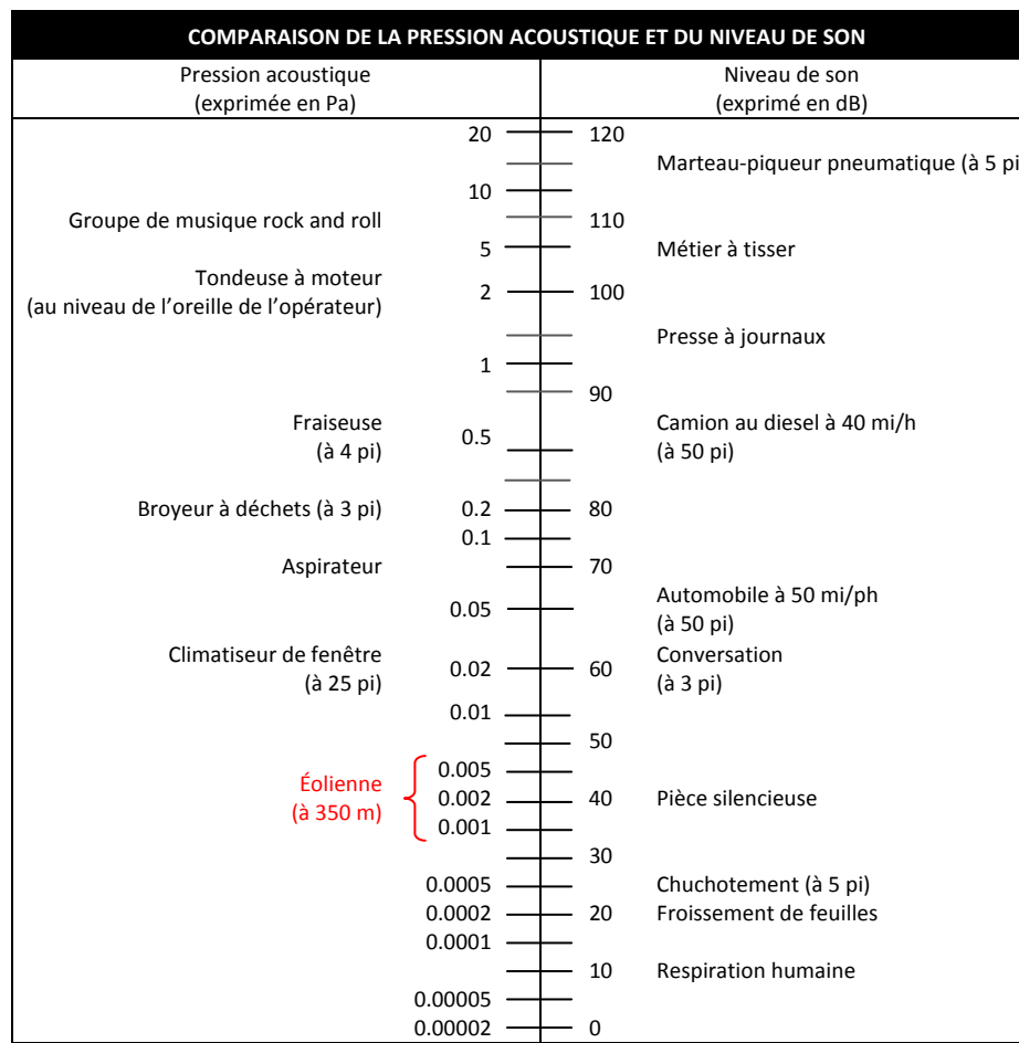
Figure 2. Comparaison de la pression acoustique (exprimée en Pa) et du niveau de son (exprimé en dB) (d'une éolienne par rapport à d'autres sources)
